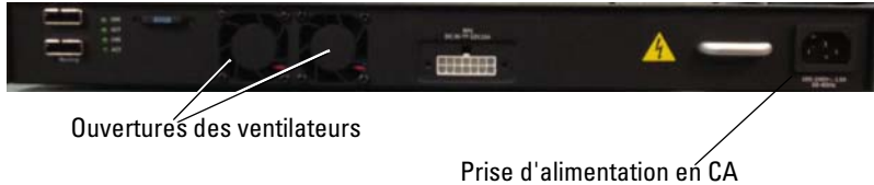
Figure 1-4. Panneau arrière N20xx
