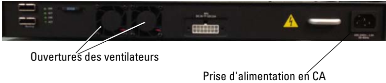
Figure 1-4. Panneau arrière N20xx
