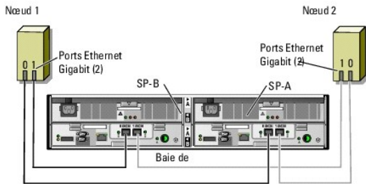
Figure 2-5. Câblage reliant un cluster à deux nœuds à un système de stockage AX4-5i
