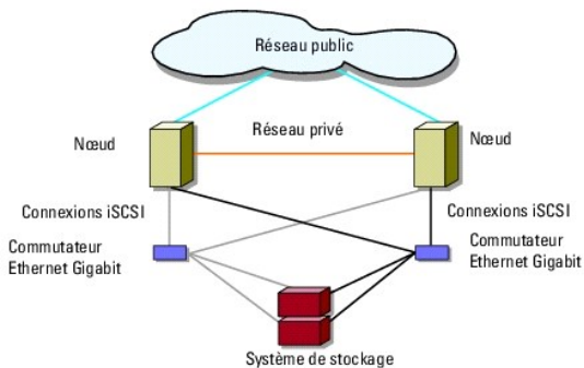
Figure 2-7. Cluster iSCSI de 8 nœuds connecté à un SAN
