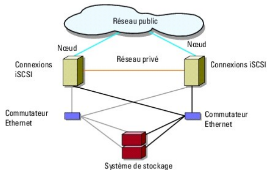
Figure 1-2. Cluster iSCSI connecté à un SAN
