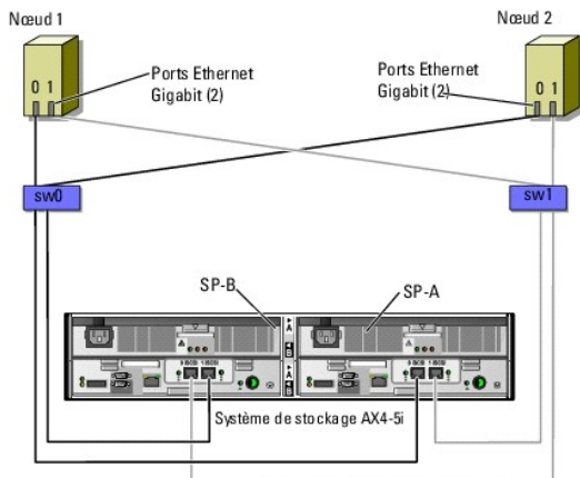
Figure 2-8. Raccordement d'un cluster iSCSI avec connexion à un SAN et du Dell|EMC AX4-5i
