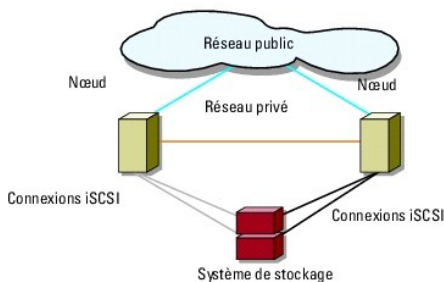
Figure 2-4. Configuration d'un cluster à connexion directe
