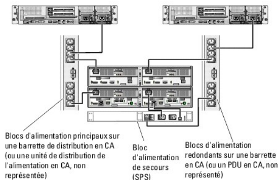
Figure 2-1. Exemple de câblage de l'alimentation comprenant un bloc d'alimentation dans les systèmes PowerEdge et un bloc d'alimentation de secours SPS dans la baie de stockage AX4-5i
