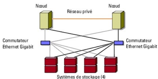
Figure 2-9. nœuds de cluster PowerEdge reliés à quatre systèmes de stockage
