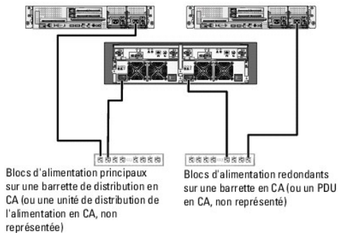
Figure 2-1. Exemple de câblage avec un module d'alimentation dans les systèmes PowerEdge
