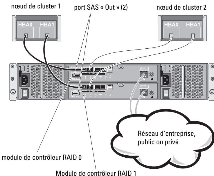
Figure 2-4. Raccordement d'un cluster de deux nœuds à connexion directe à un système de stockage PowerVault MD36x0f
