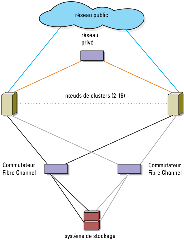
Figure 2-7. Cluster de 16 nœuds connecté à un SAN
