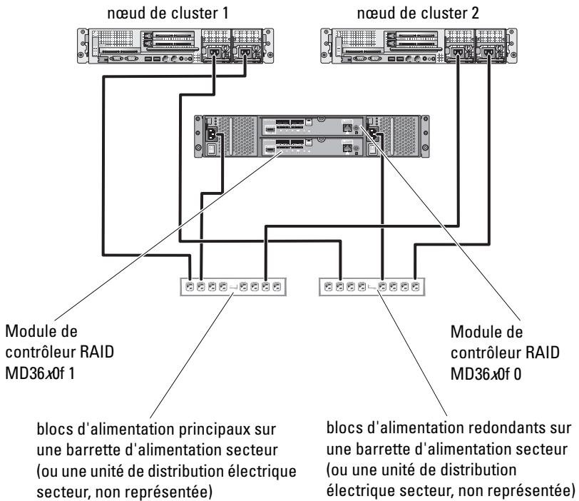
Figure 2-1. Exemple de câblage électrique
