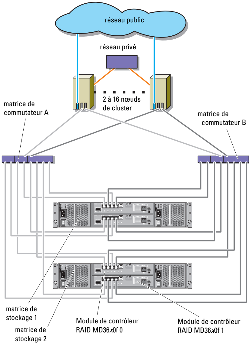
Figure 2-10. Configuration d'un cluster avec connexion à un SAN incluant plusieurs matrices de stockage
