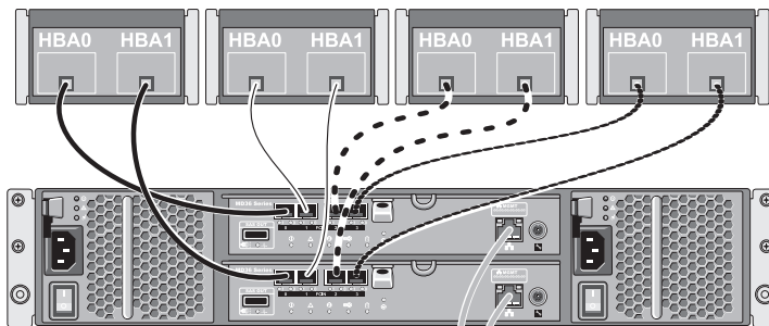
Figure 2-5. Raccordement d'un cluster de quatre nœuds à connexion directe à un système de stockage PowerVault MD36x0f
