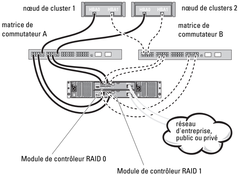
Figure 2-8. Câblage reliant un cluster connecté à un SAN à MD36x0f
