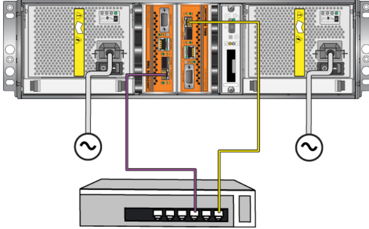
Şekil 3-9: Minimum Ağ Yapılandırması
