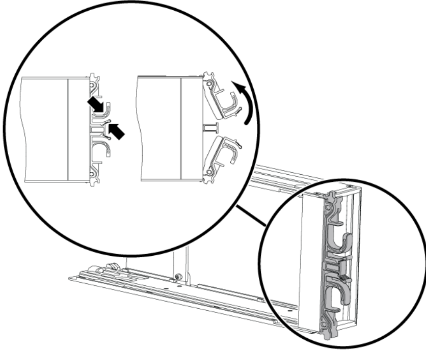
Şekil 3-2: Bir Kontrol Modülü Mandalının Açılması
