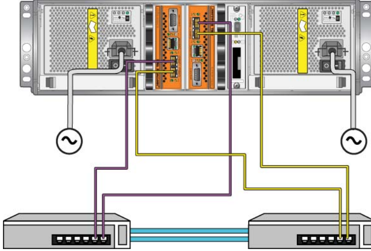
Şekil 3-10: Yönetim Ağı Olmadan Yapılandırma
