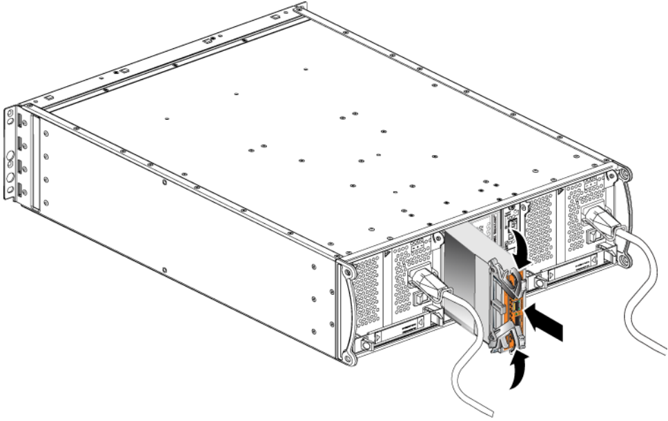
Şekil 3-5: Bir Kontrol Modülünün Takılması
