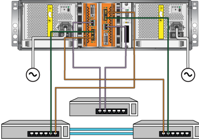
Şekil 3-11: Yönetim Ağı İle Yapılandırma
