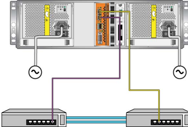
Şekil 3-8: Tavsiye edilen Tek Kontrol Modülü Yapılandırması
