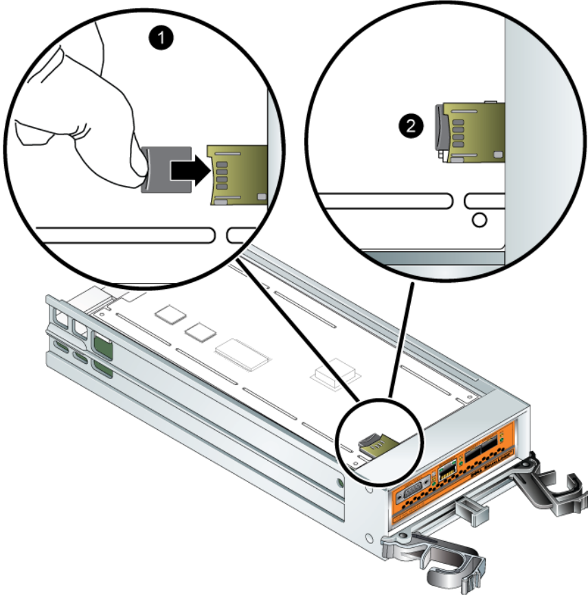
Şekil 3-7: Mikro SD Kartının Takılması
