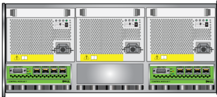
Şekil 2-10: PS6500 Dizi - Arkadan Görünüş
