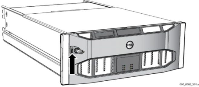
Şekil 2-20: Çerçeve Serbest Bırakma Mandalını İtme
