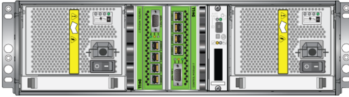
Şekil 2-3: PS6000 Dizi - Arkadan Görünüş
