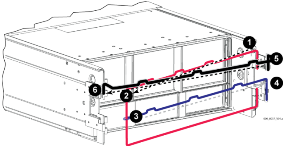
图 2-14: 电缆布线图
