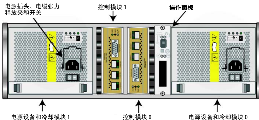
图 1-2:PS5000 背面板
