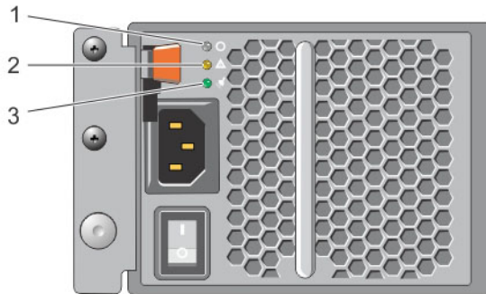
Ilustración 8. LED e interruptor de alimentación de CA
