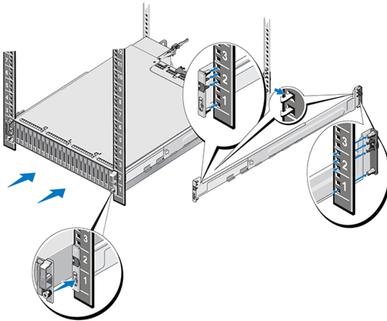
图 2: 将阵列安装到机架中
