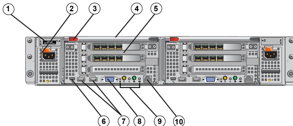
그림 4: 후면 패널
