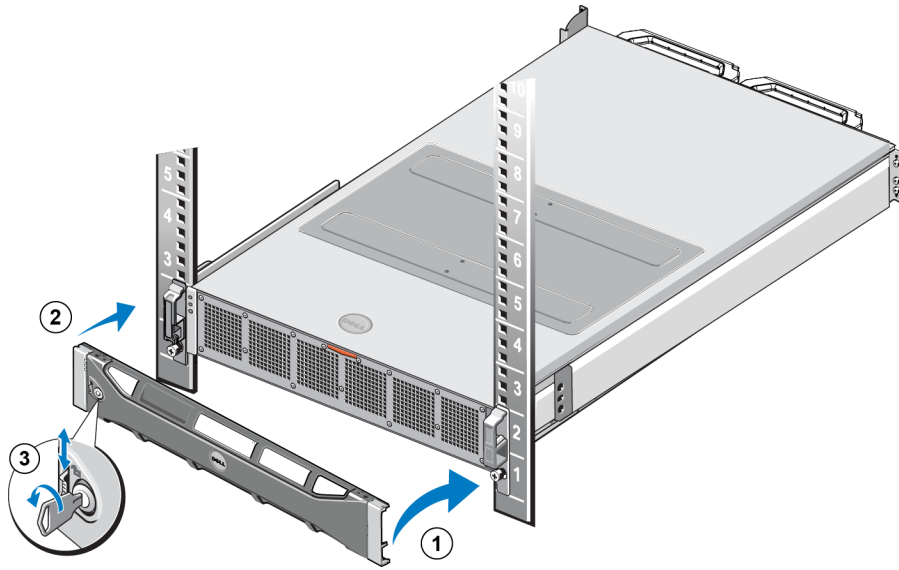
그림 6: 베젤 장착
