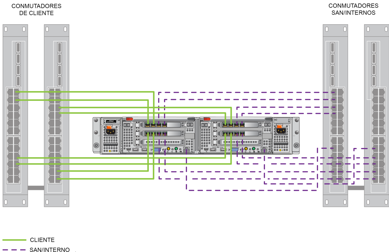
Ilustración 9: Configuración de red de EqualLogic FS7600
