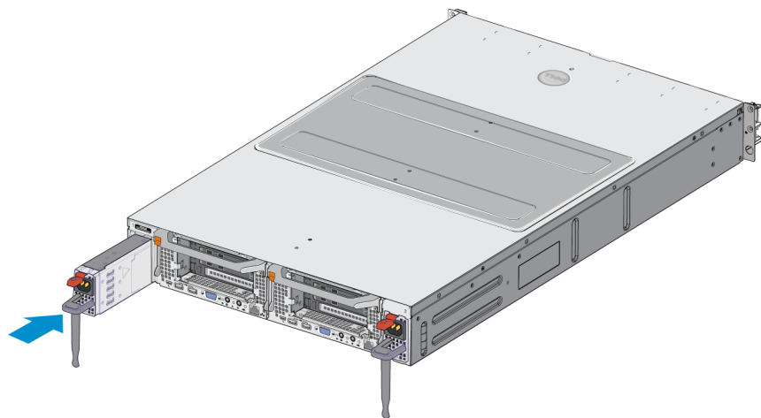
Рис. 10: Установка блока питания
