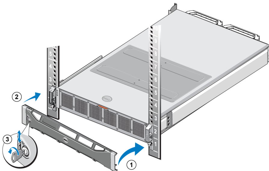
Рис. 12: Крепление лицевой панели
