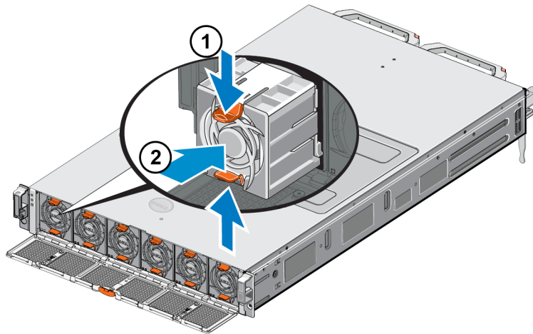
Рис. 15: Установка охлаждающего вентилятора
