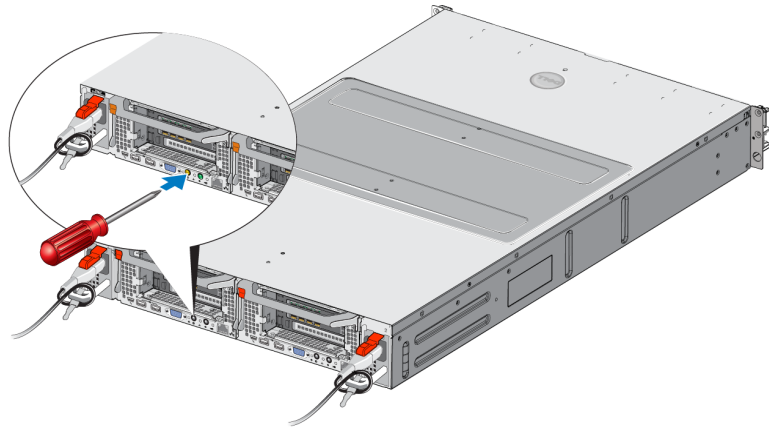
Рис. 5: Включение и выключение питания контроллера
