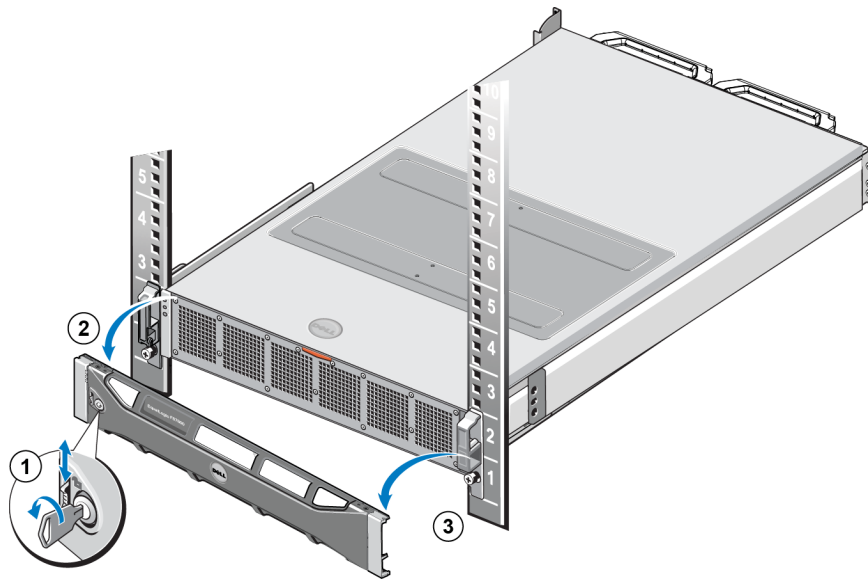
Рис. 11: Снятие лицевой панели
