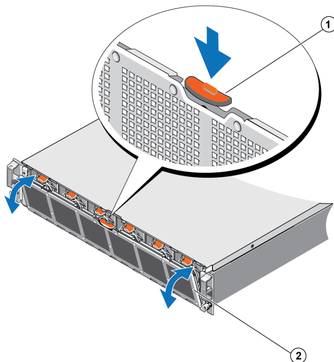
Рис. 13: Открытие и закрытие смотровой дверцы вентилятора
