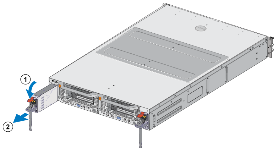
Рис. 9: Извлечение блока питания
