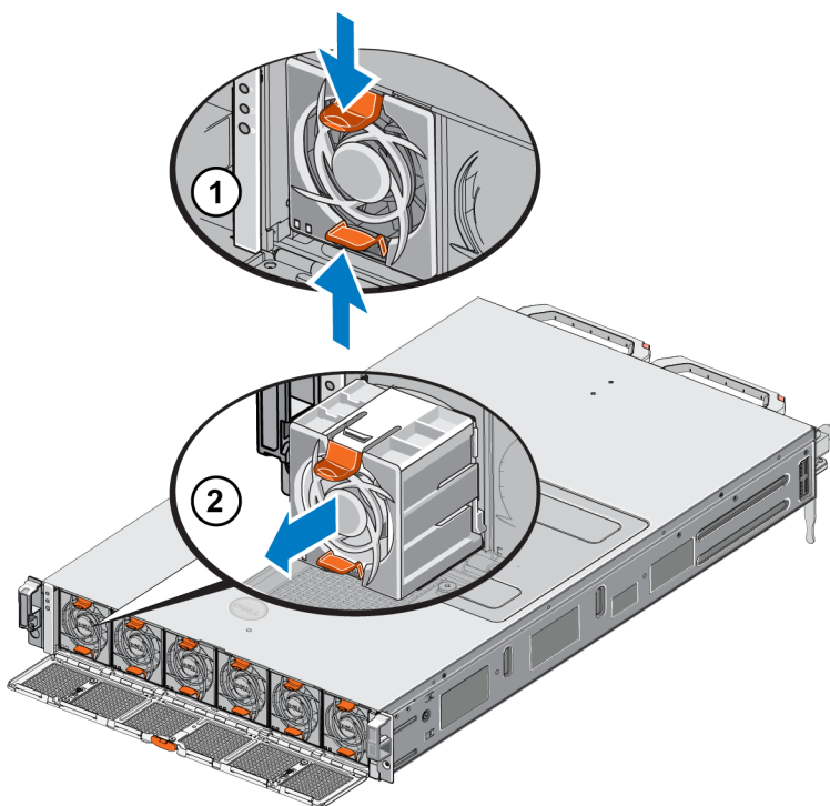
Рис. 14: Извлечение вентилятора
