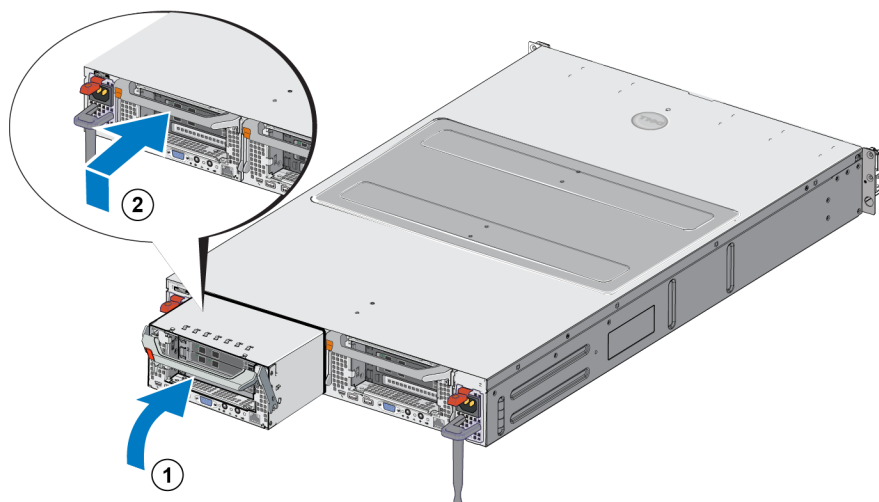
Рис. 8: Установка контроллера
