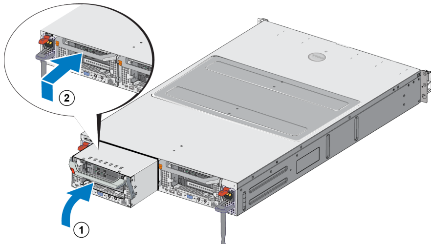
그림 8: 컨트롤러 설치
