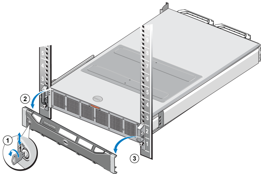
그림 11: 베젤 분리
