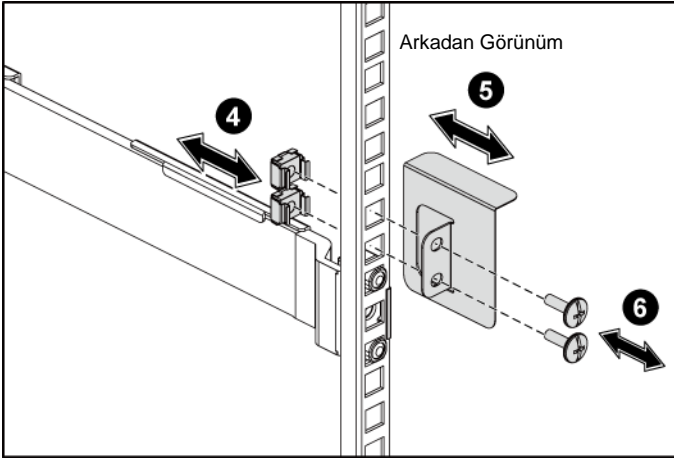
Şekil 3. Kasa Dengeleyici Nakliye Braketlerini Takma
