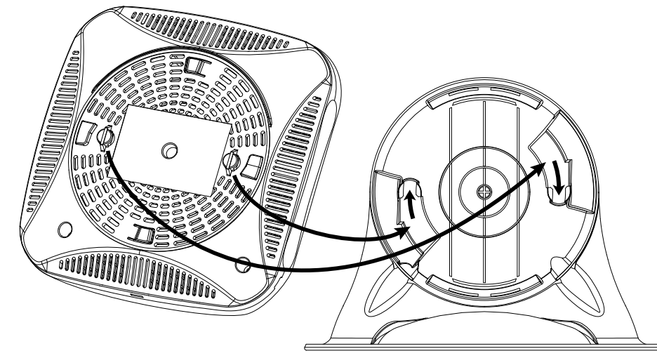
Figura 3 Instalación vertical
