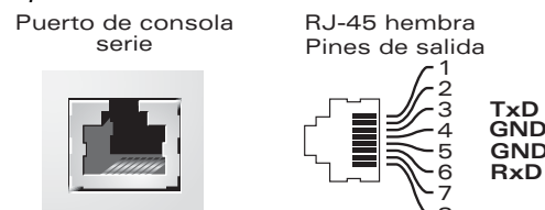
Figura 4 Pines del puerto serie
