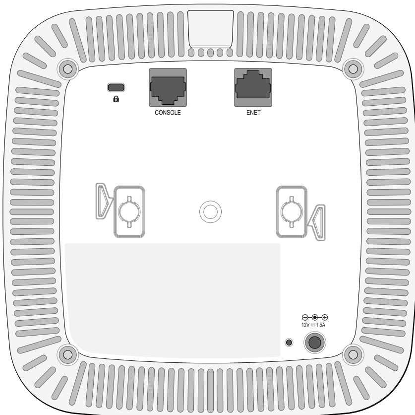
Figura 3 Vista posterior del Serie W-AP110
