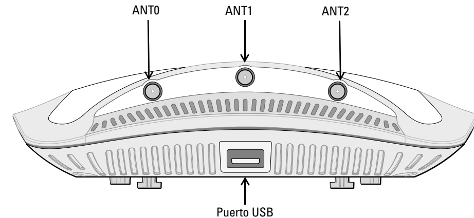
Figura 2 Vista lateral del Serie W-AP110 (W-AP114 mostrada)
