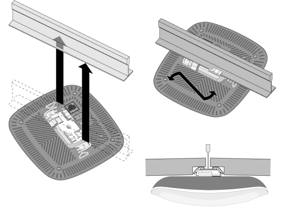
圖 5 安裝 AP
