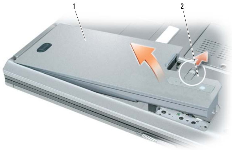
1 电池 2 电池槽释放门锁
