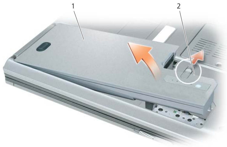
1 バッテリー 2 バッテリーベイリリースラッチ
