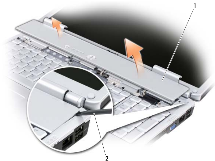
1 cache de la charnière 2 pointe en plastique
