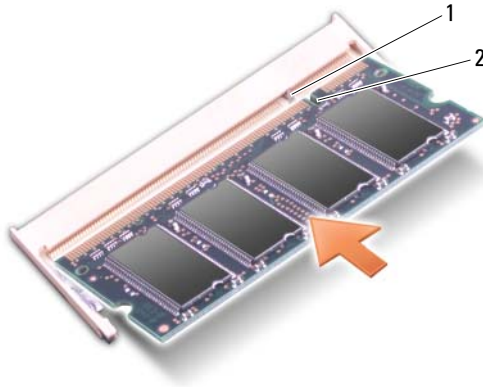
1 languette 2 encoche
