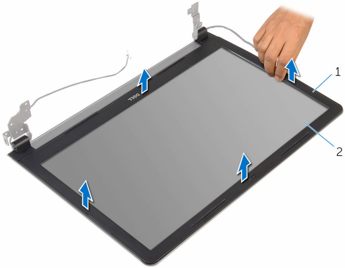
1 display bezel
