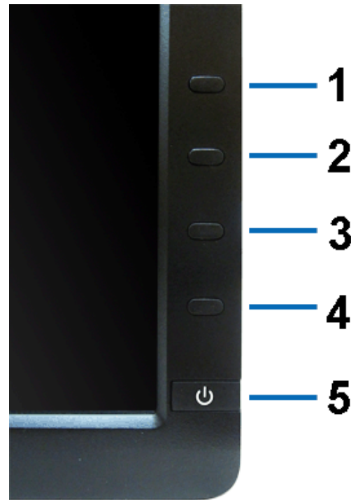
Bedienelemente an der Vorderseite
