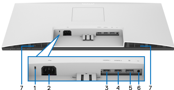
底视图（无显示器支架）
