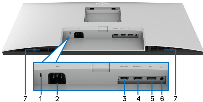
底视图（无显示器支架）
