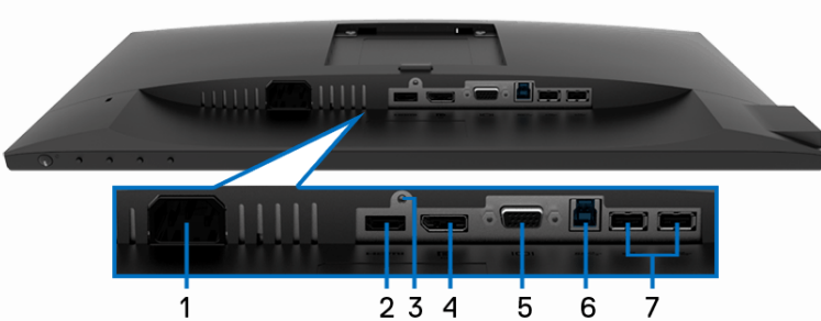
Ansicht von unten ohne Monitor-Standfuß
