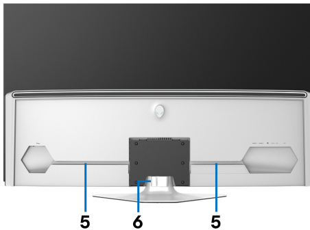
Vue arrière avec pied du moniteur
