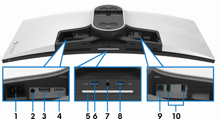
無顯示器支架的後視圖和底視圖
