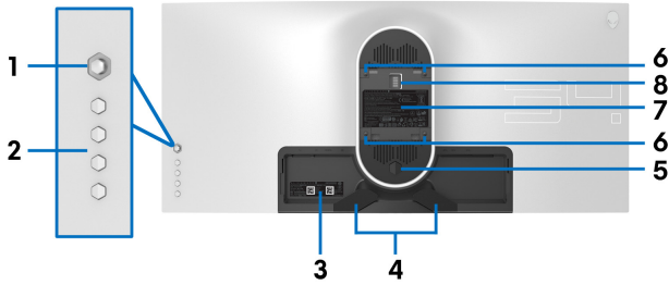
모니터 스탠드 미장착 상태의 뒷면
