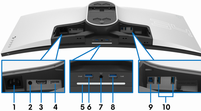
후면 및 밑면 모습 (모니터 스탠드 없음)
