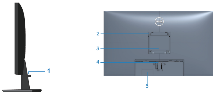
モニタースタンドを取り付けた状態の背面ビュー
