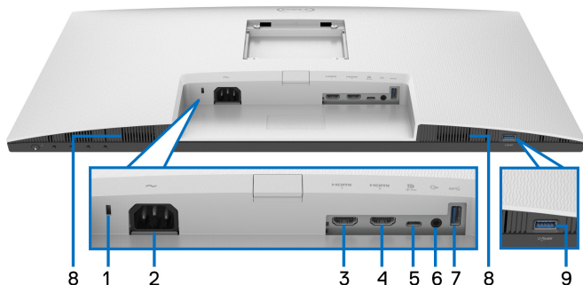
Вигляд знизу без стійки монітора
