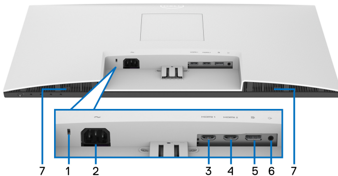
Κάτω πλευρά χωρίς το στήριγμα οθόνης
