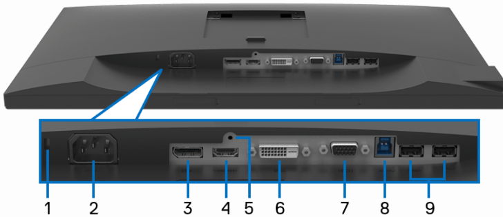
底视图（无显示器支架）
