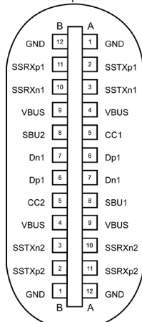
USB Type-C receptacle
