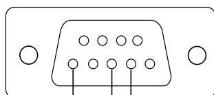
公头 GND TXD RXD
