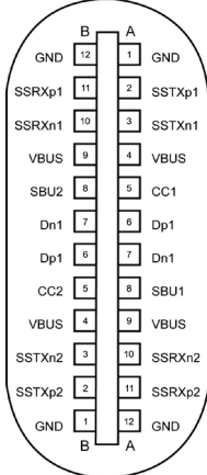
USB Type-C foglalat
