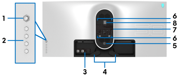
Ansicht von hinten ohne Monitor-Standfuß
