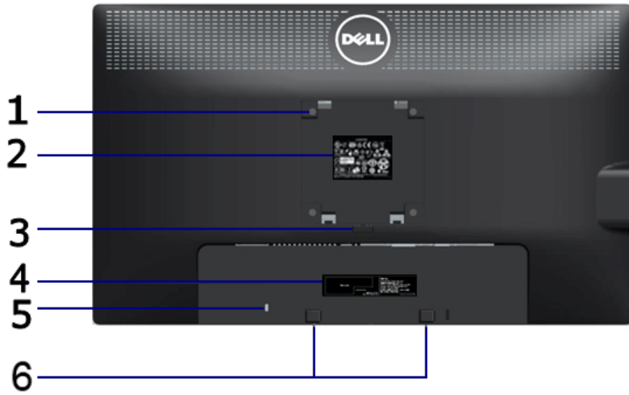
后视图
