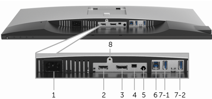
底视图（无显示器支架）
