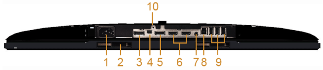
منظر سفلي بدون حامل شاشة
