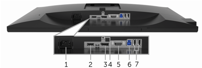
底视图（无显示器支架）
