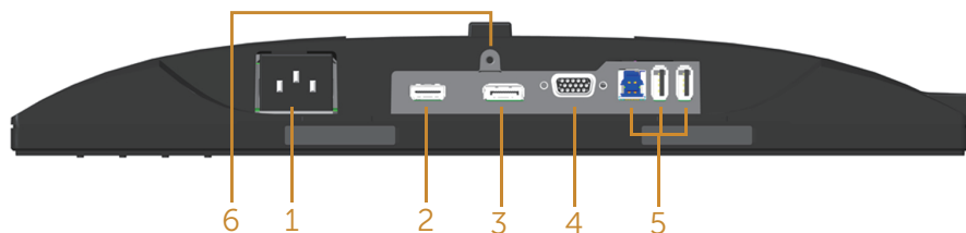
モニタースタンドを取り付けていない状態の底面ビュー
