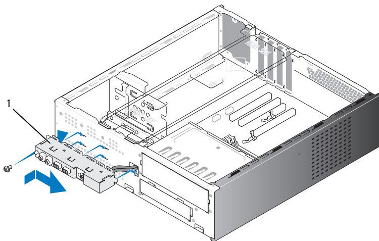
1 I/O パネル
