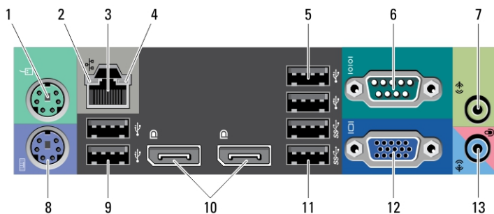
圖 3. 迷你直立型電腦和桌上型電腦的背面板視圖
