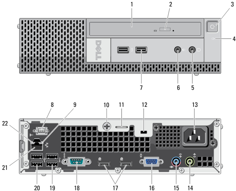
圖 6. 超小型電腦的前視圖與後視圖
