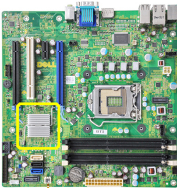
Angka 1. Board Sistem dari versi terdahulu dari board sistem dengan unit pendingin
