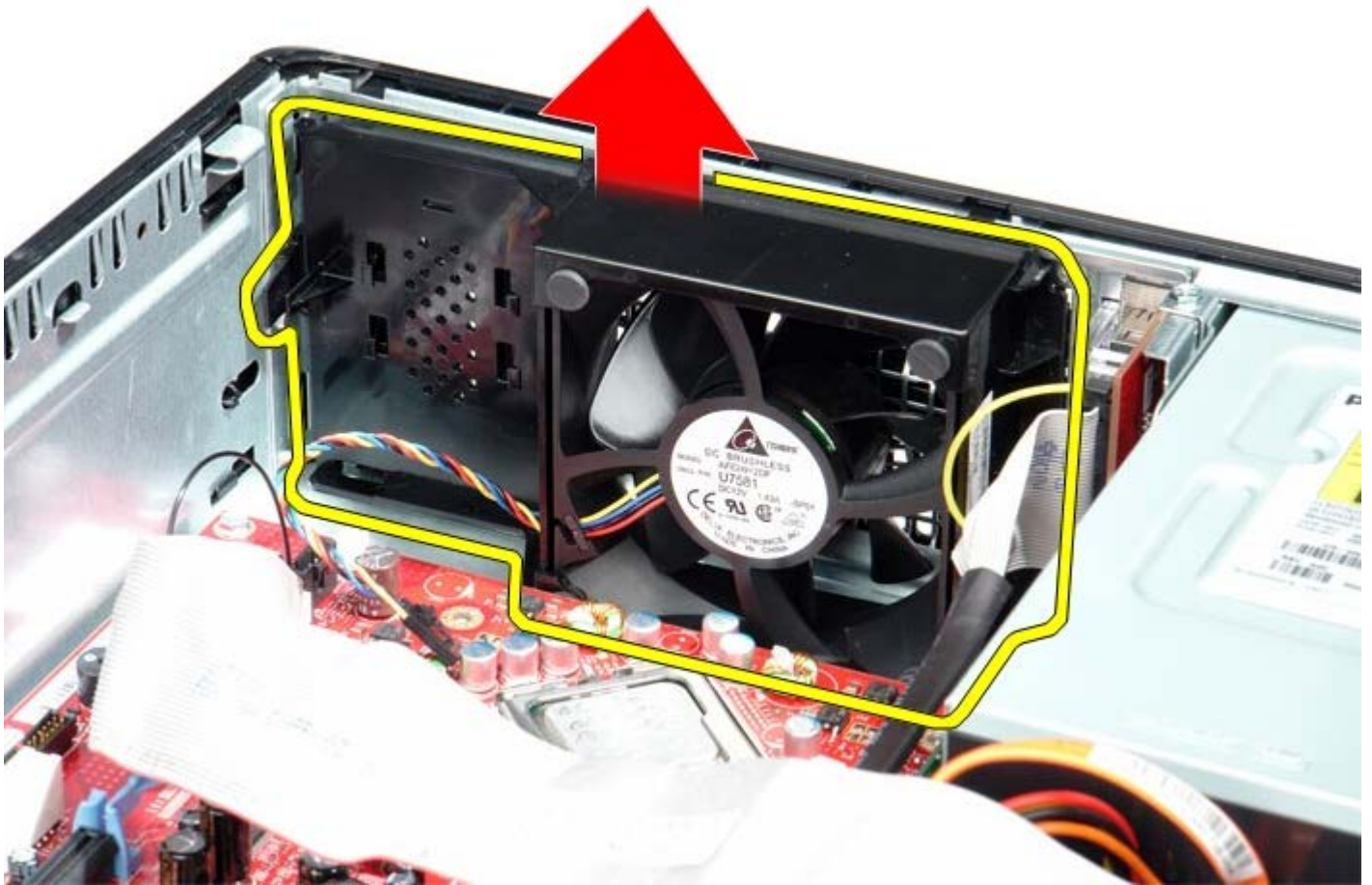
1 11 提起风扇并将其从计算机中卸下。
