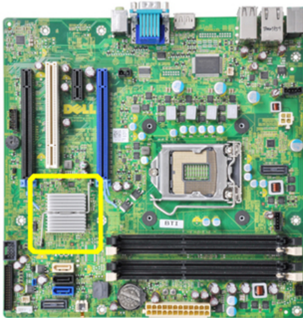
Figura 1. Placa de sistema de uma versão anterior com dissipador de calor
