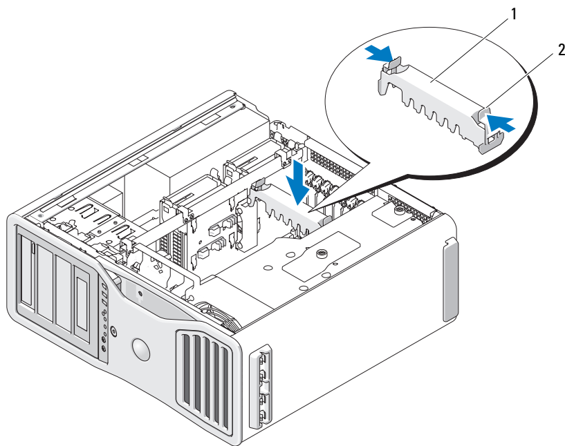
1 держатель платы 2 фиксатор
