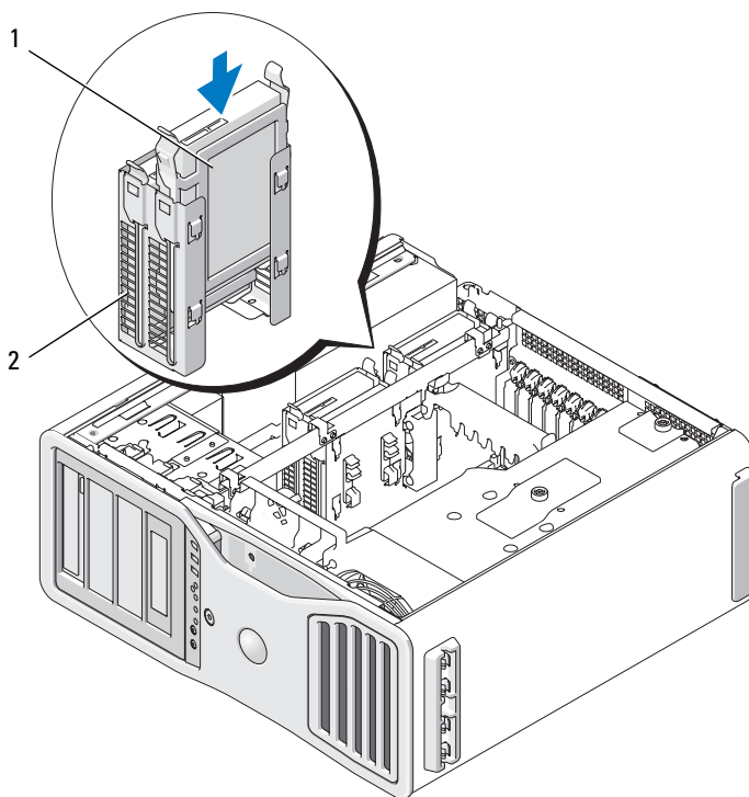
1 жесткий диск 2 отсек жесткого диска
