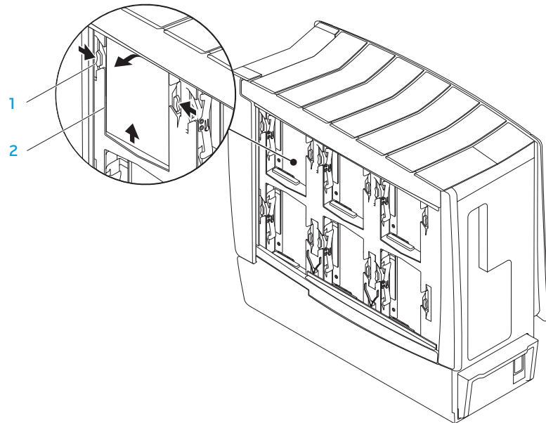
1 釋放夾 (2 個)
