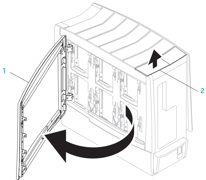
2 釋放面板
