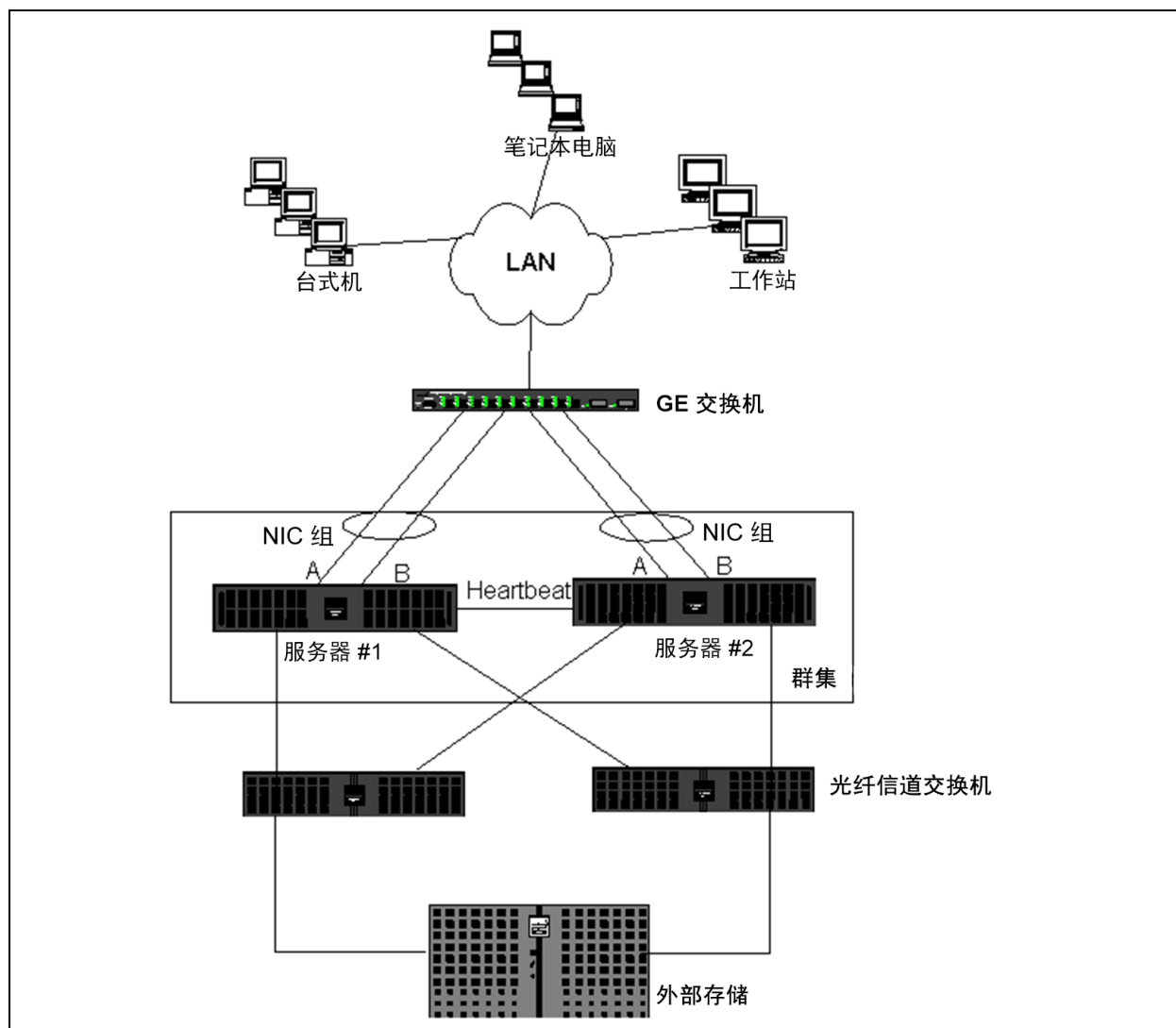
图 11-7. 跨一台交换机组合的群集
