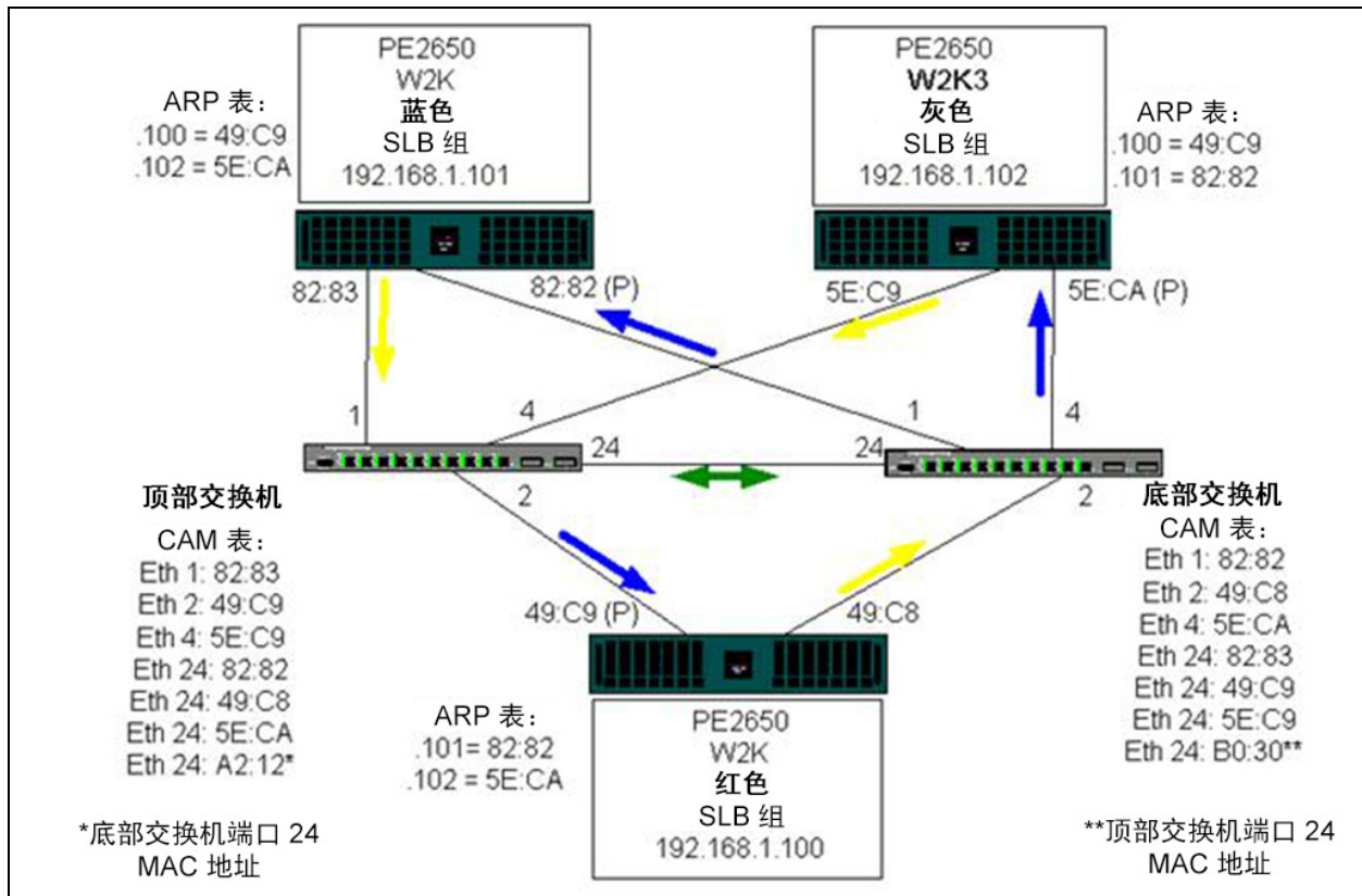
图 11-4. 在互相连接的情况下跨交换机组合
